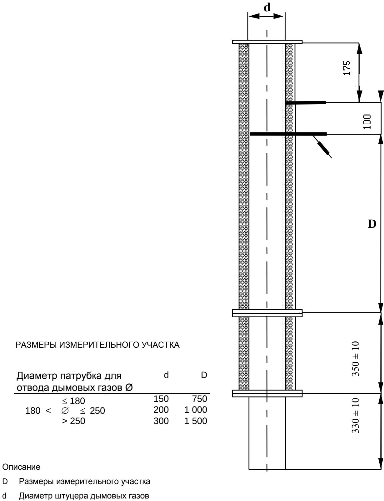
Рисунок А.9 — Детали и размеры измерительного участка с вертикальным штуцером отвода дымовых газов
