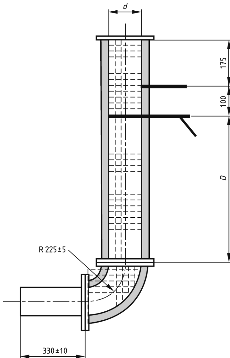
Размеры измерительного участка
