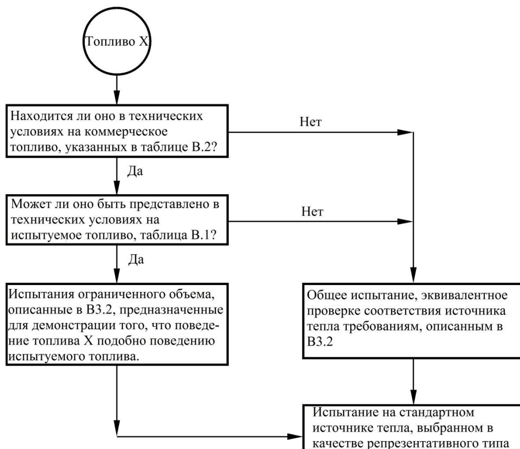
Рисунок В.1 — Схема процесса выбора топлива, рекомендуемого для испытаний
