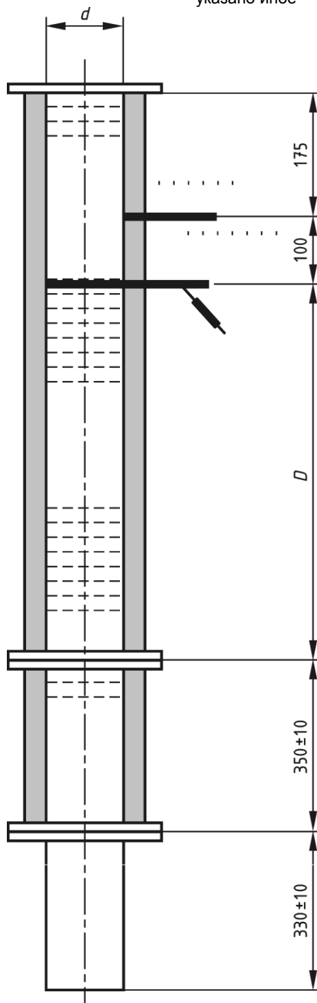
Размеры измерительного участка
