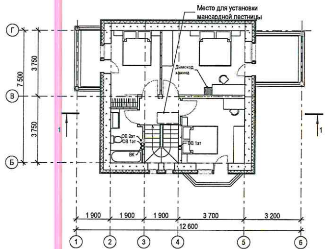
План 2 этажа
