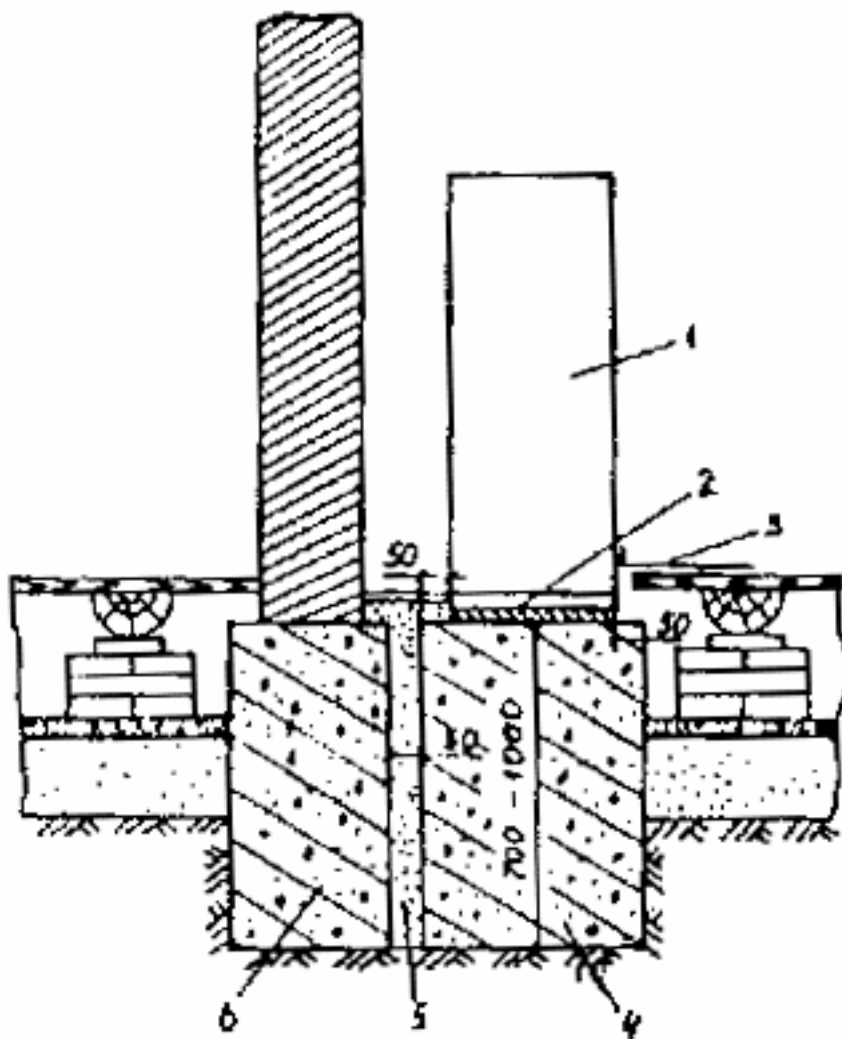
Рис. 3.2. Размещение печи на отдельном фундаменте
