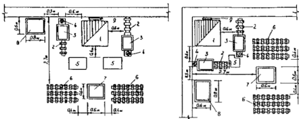
Рис. 2.1. Схема организации рабочего места при кладке печи у стены и в углу помещения
