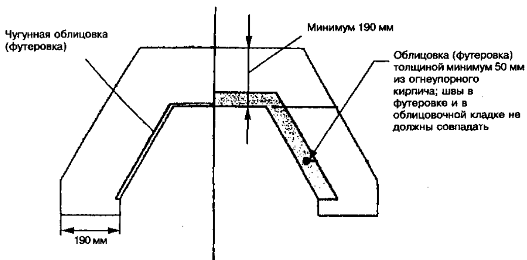
Рисунок 7.5 — Футеровка камина
