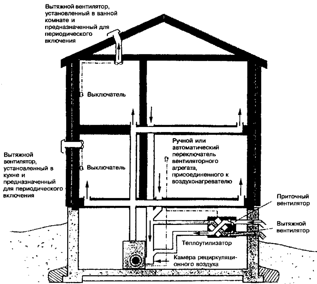
Рисунок 7.3 — Присоединение теплоутилизационного агрегата к камере подогрева воздуха
