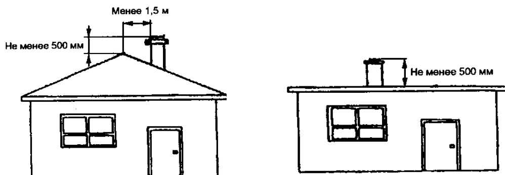
Рисунок 7.8 — Расстояние от дымовой трубы до строительных конструкций
