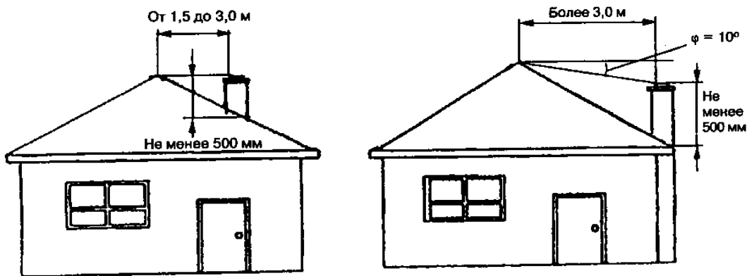
Рисунок 7.9— Минимальная высота дымовой трубы
