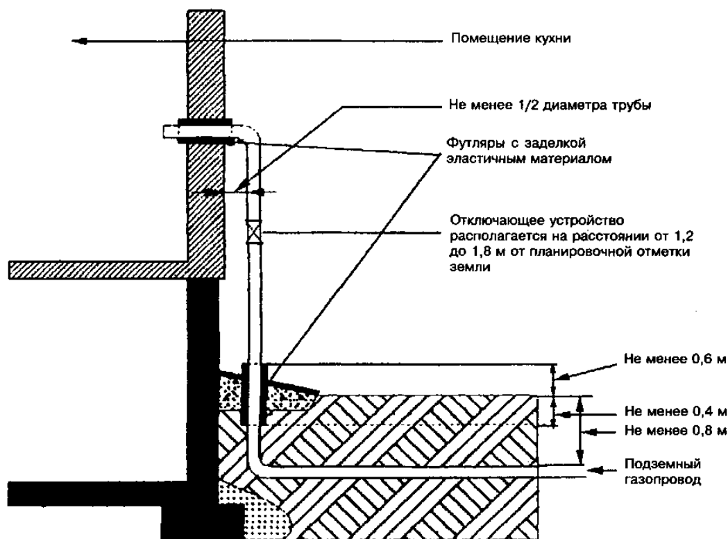
Рисунок 9.1 — Газовый ввод
