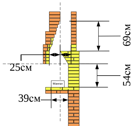
Вид с боку разрез
