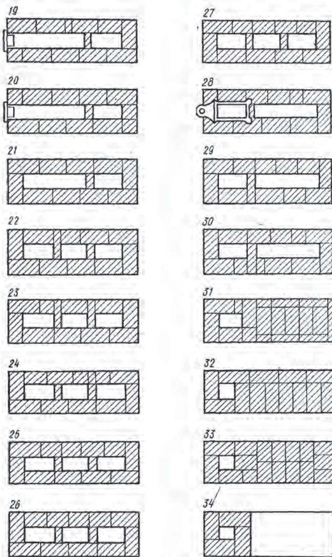
Рис. 48, б. Отопительный щиток. Ряды 19—34
