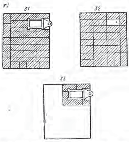
Рис. 47, ж. Печь конструкции И. Ф. Волкова. Ряды 31—33 12. Отопительный щиток к кухонной плите
